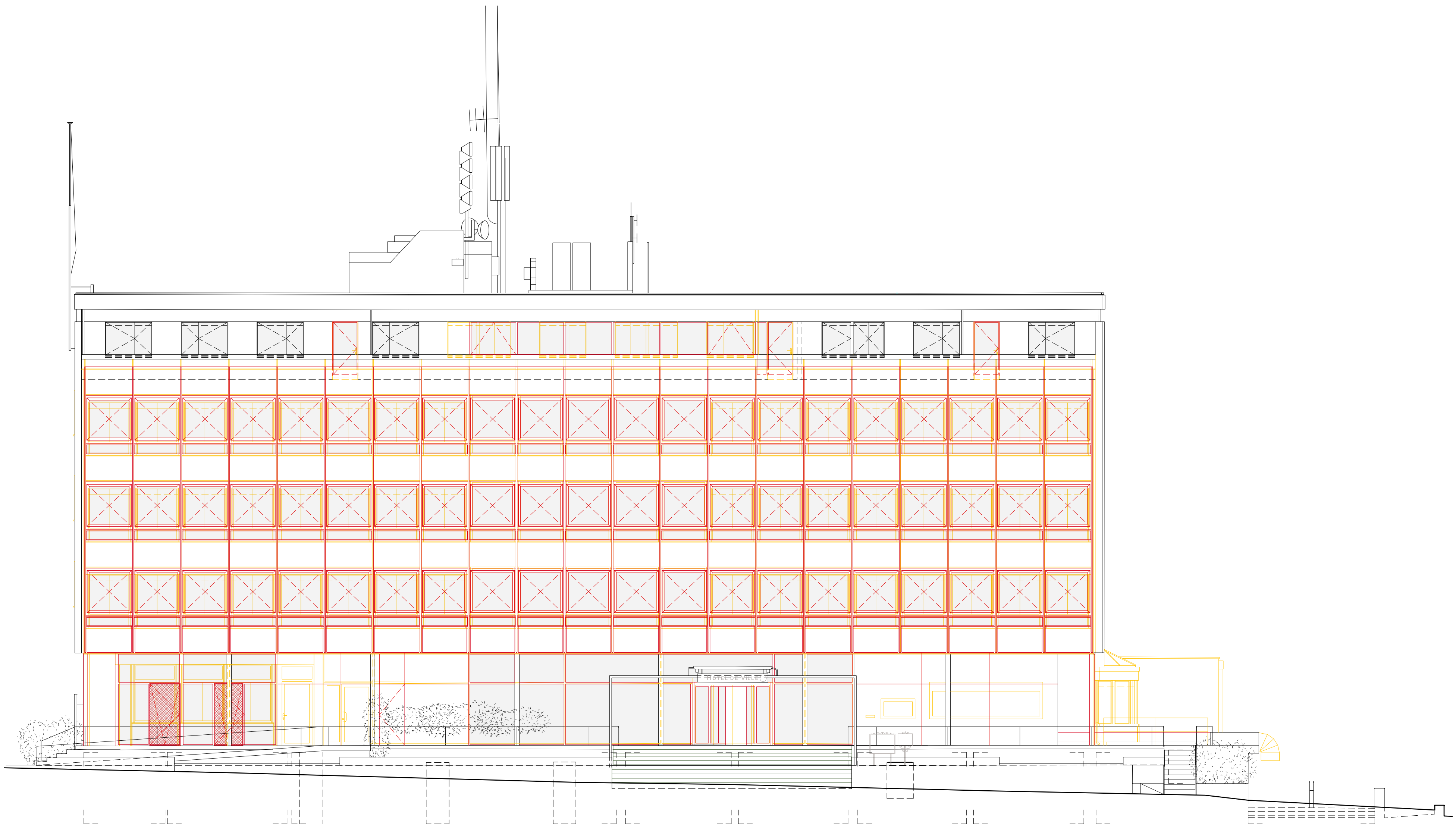
BÂTIMENT A - FACADE NORD
