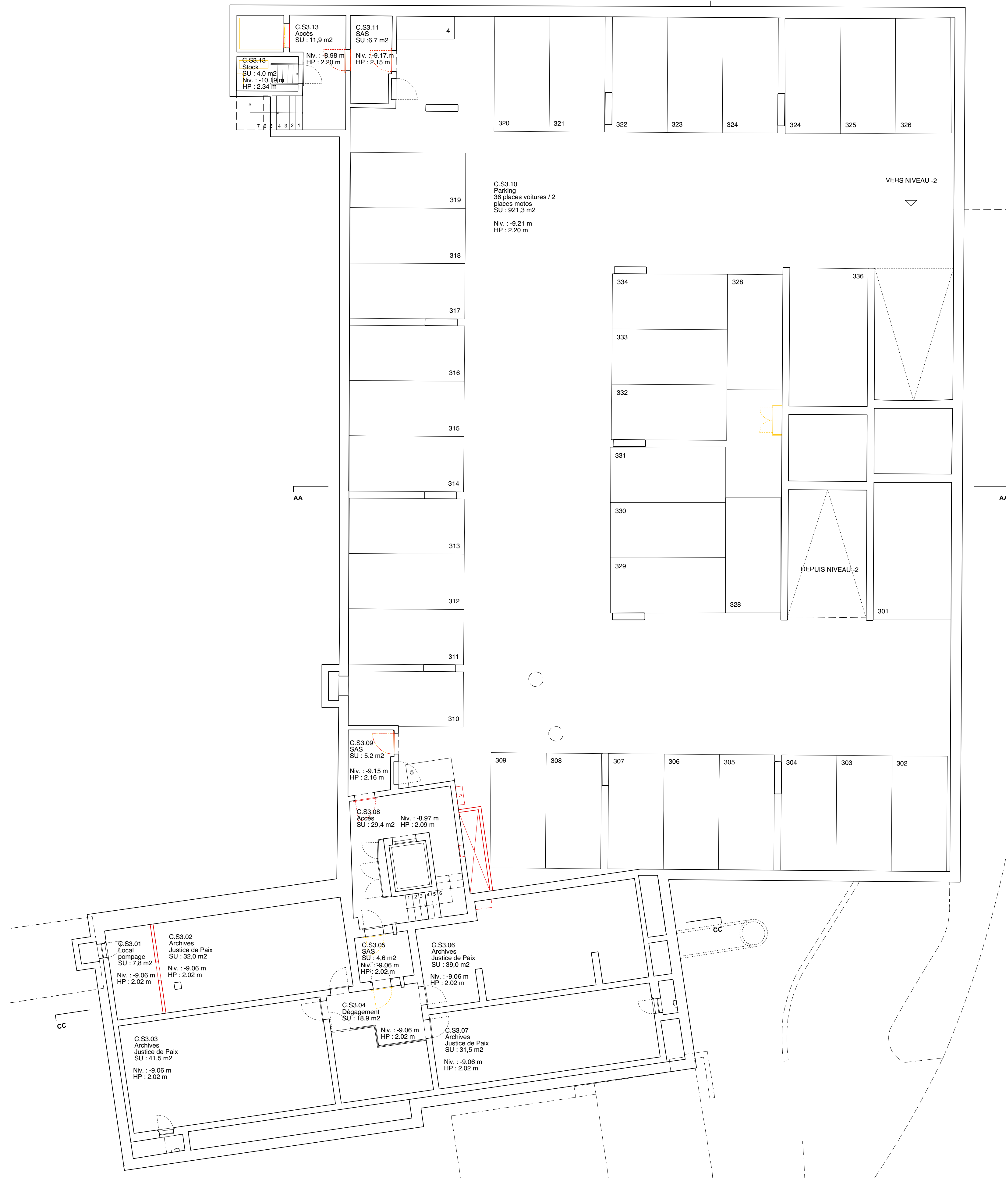
BÂTIMENT C_PLAN DU TROISIEME SOUS-SOL Hauteur plan de coupe : -8.25 m
