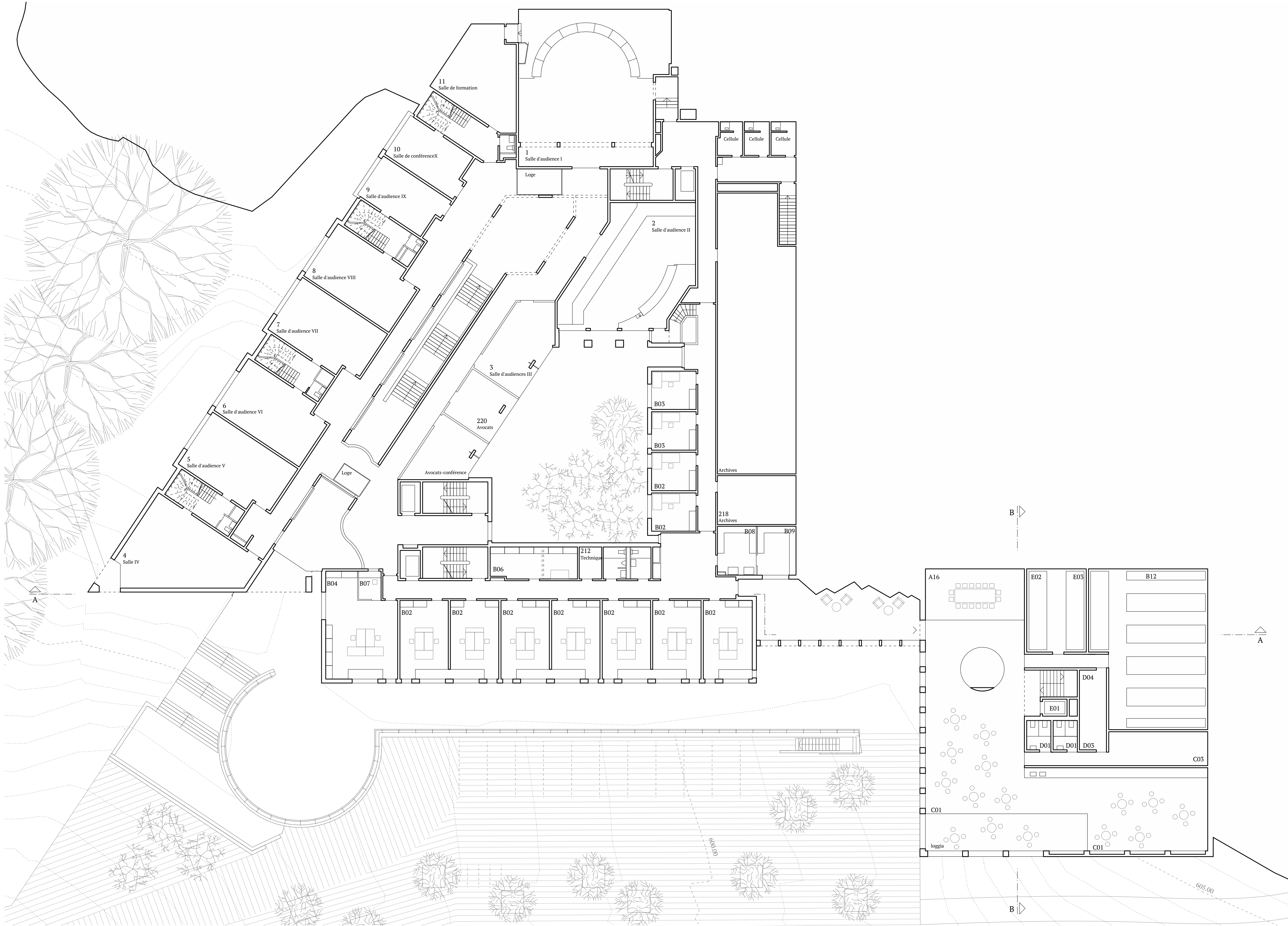
Niveau 02 _ 604.60 : C COMMUNS + LIAISON. Ech 1/200
